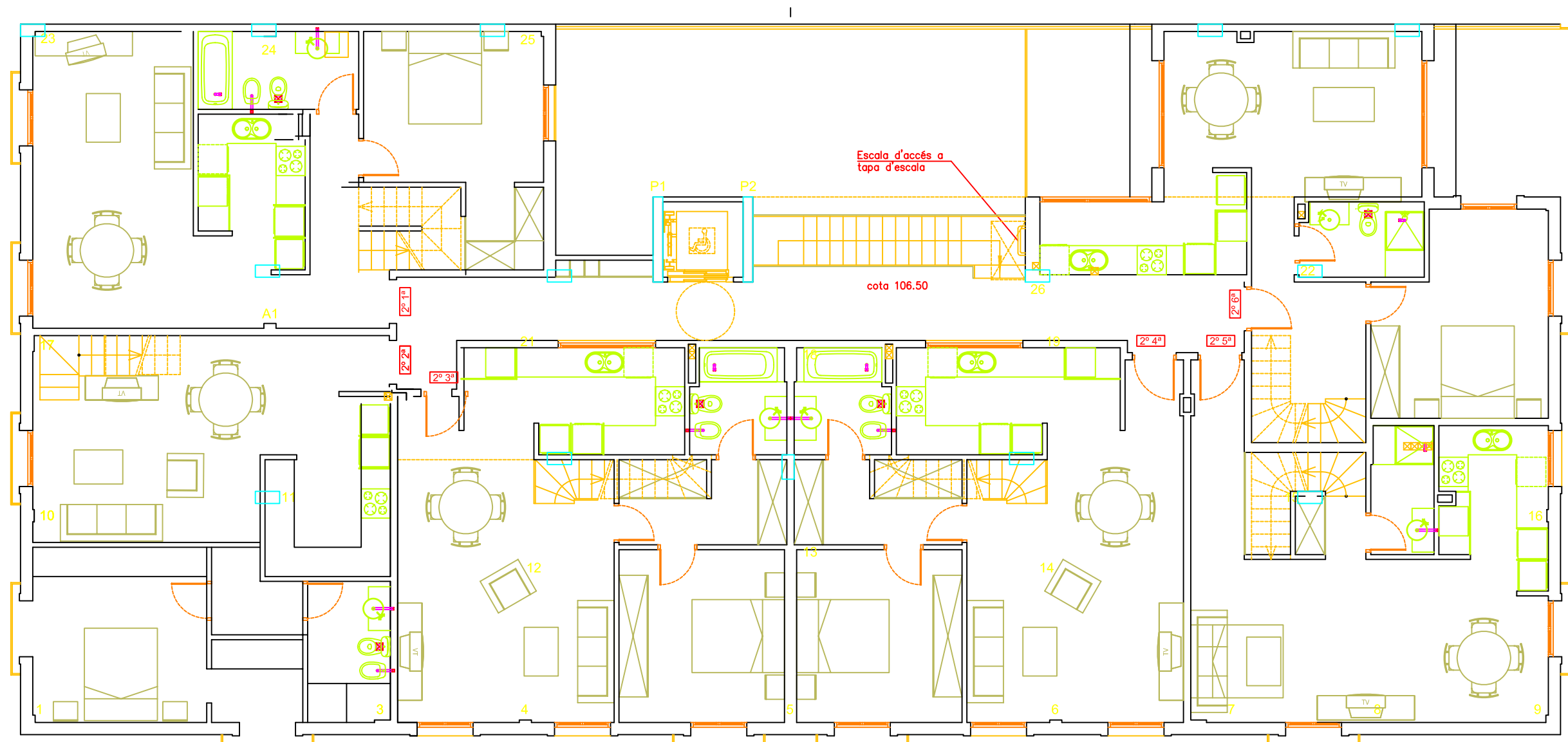
planta 2on pis
