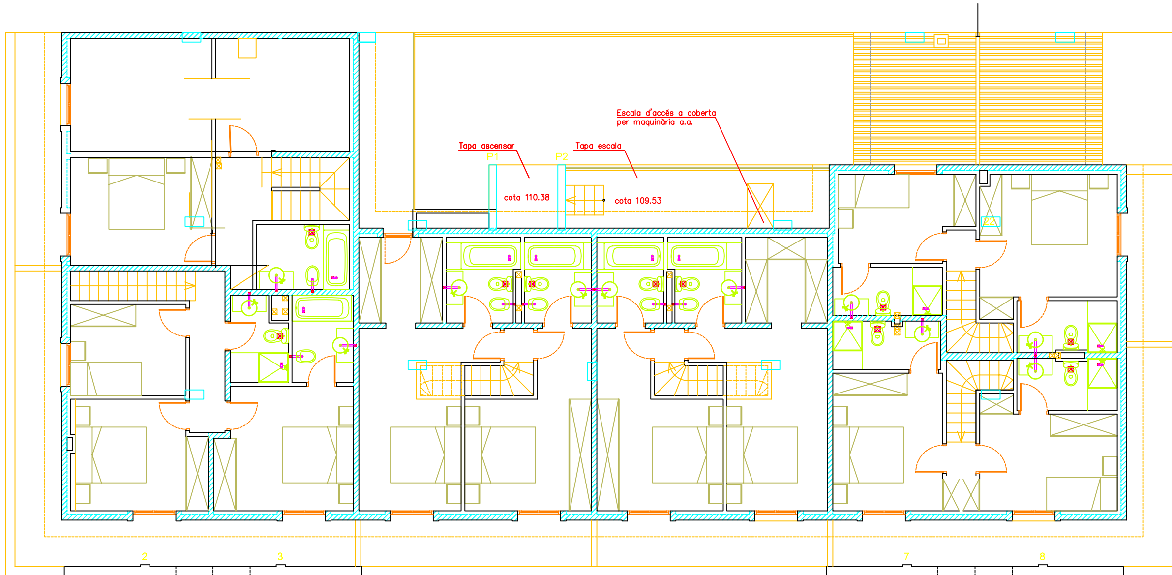
planta golfes
